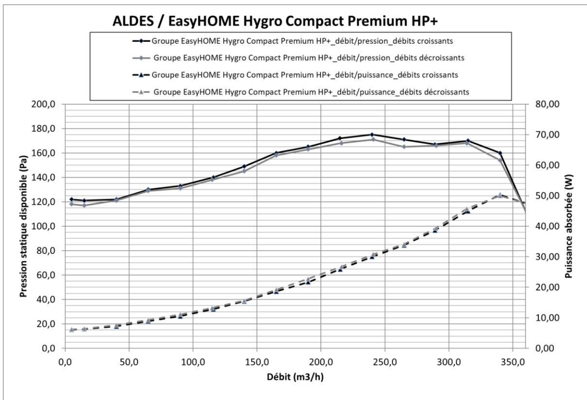
Figure 14 - Groupe d'extraction « EasyHOME Hygro COMPACT PREMIUM HP+ » - courbes caractéristiques
