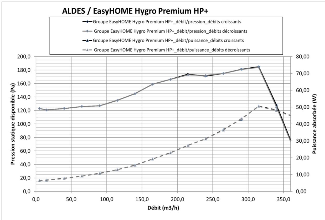
Figure 13 - Groupe d'extraction « EasyHOME Hygro PREMIUM HP+ » - courbes caractéristiques
